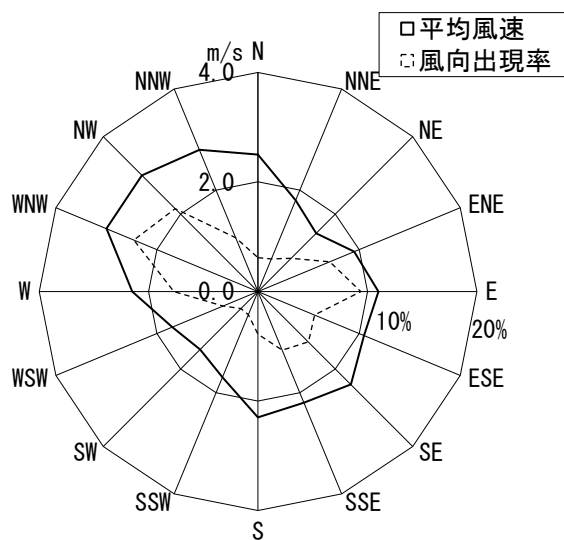
図 6.1-1 風配図 (A)
