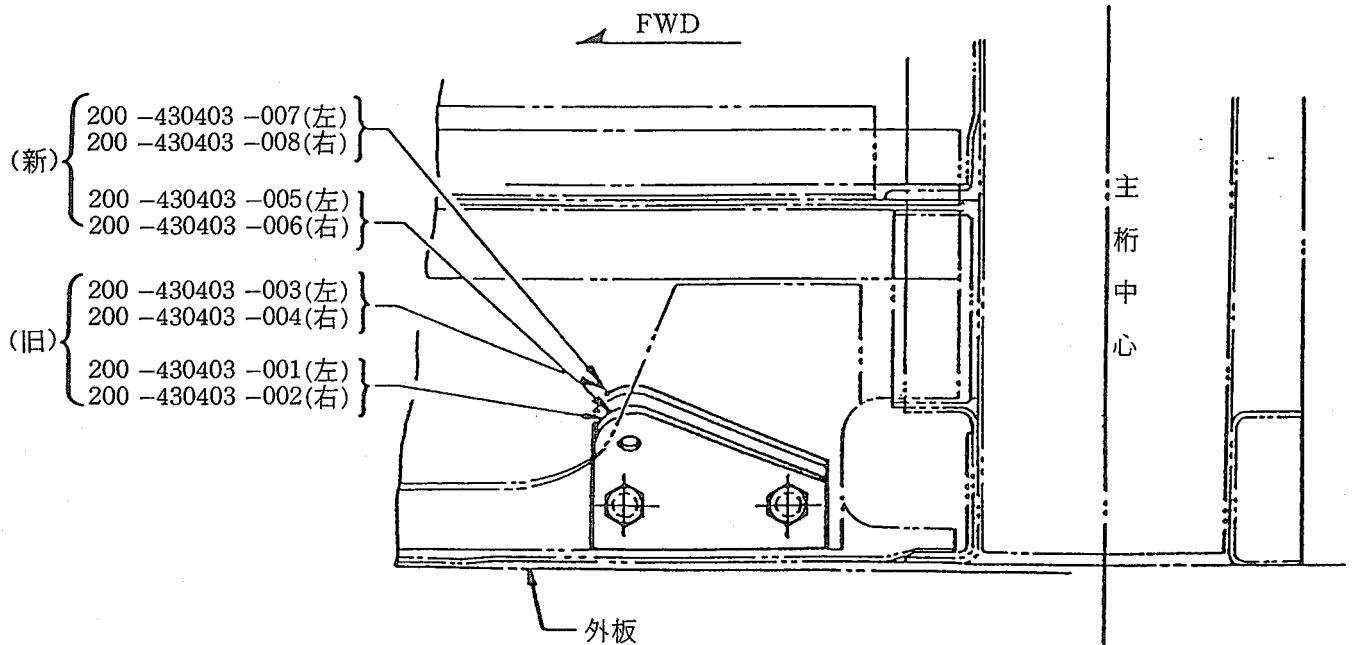
図 - 2 安全バンド取付ブラケット交換要領 (左側図示) (S/N 119 以前の機体のみ)
