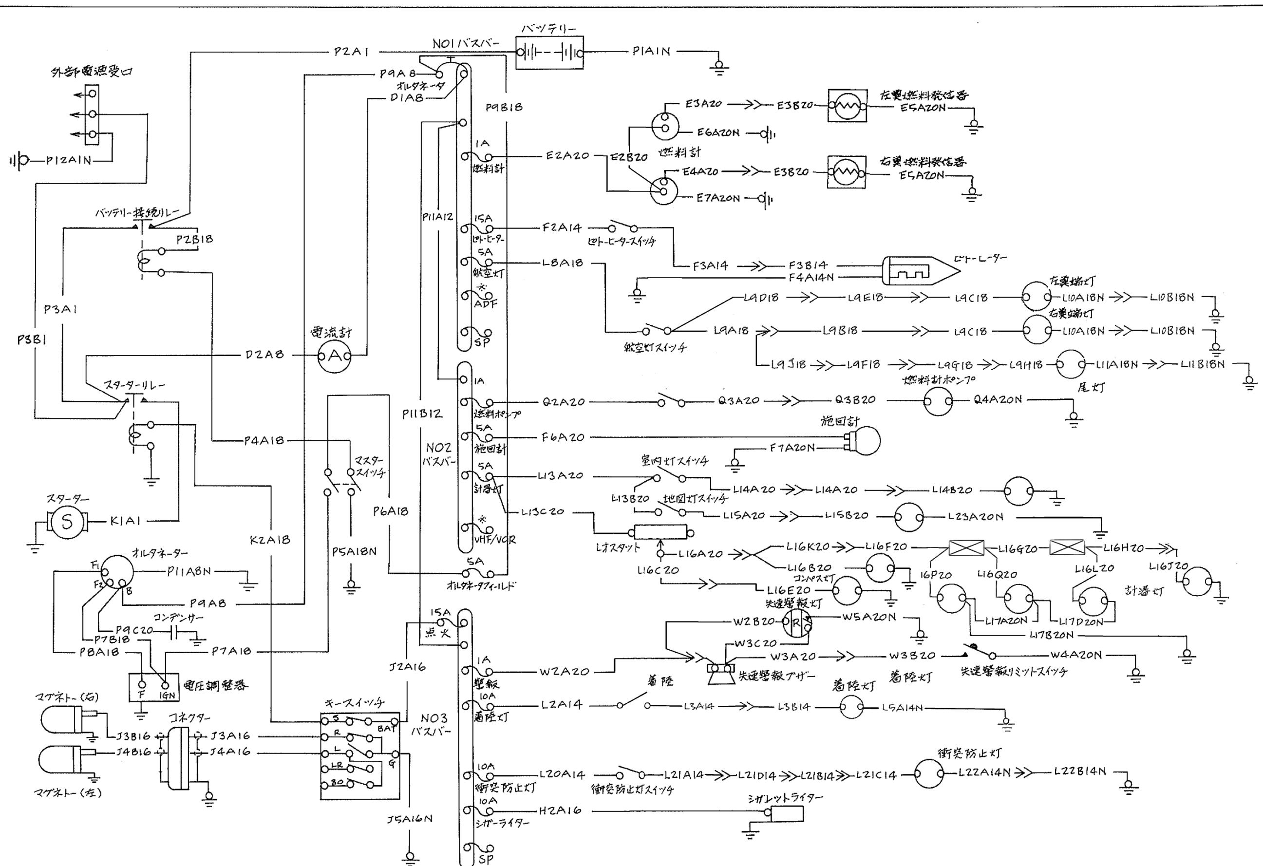
電気系統回路図
