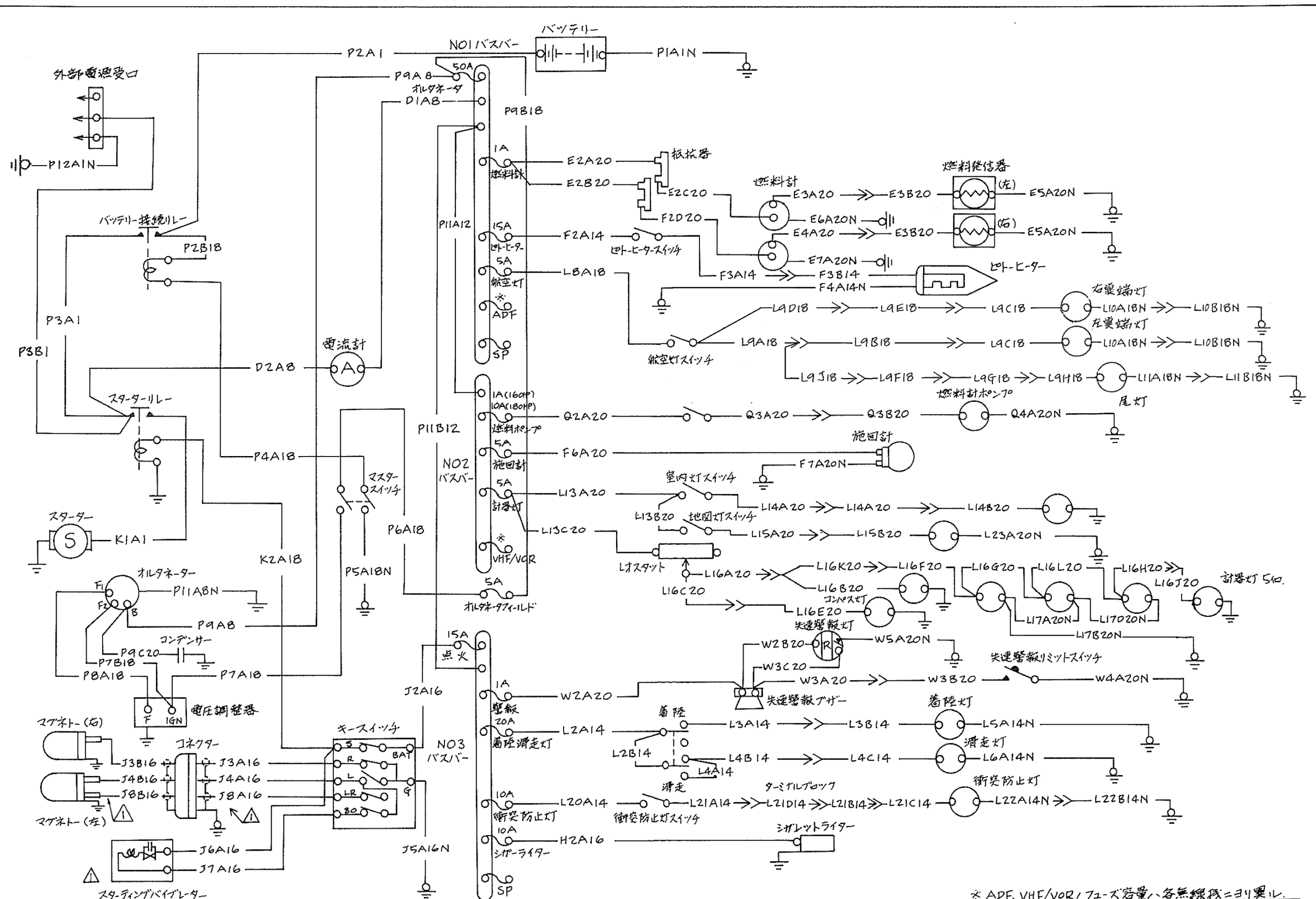
電気系統回路図
